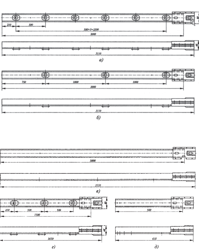
Рис. 2.2. Прямые секции шинпроводов ШОС
