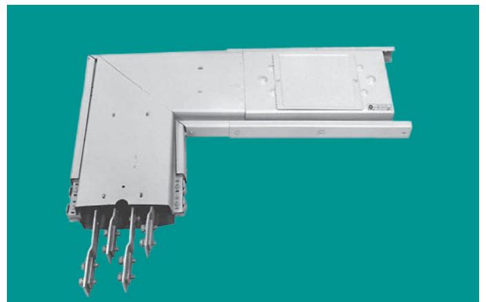
Рис. 1.9. Секции угловые горизонтальные левые
