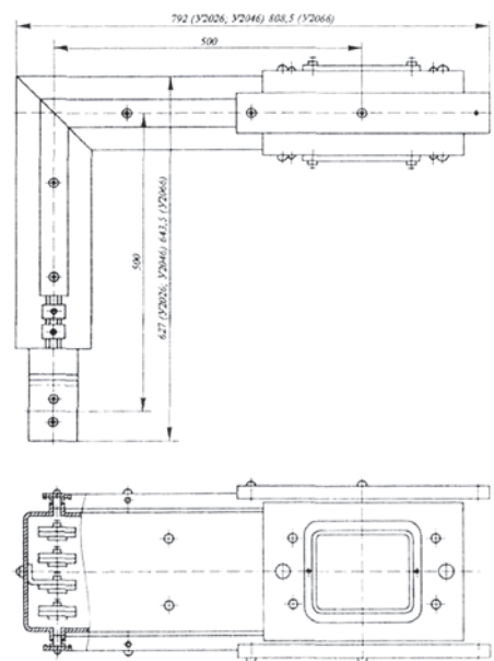
Рис. 1.9. Секции угловые горизонтальные левые
