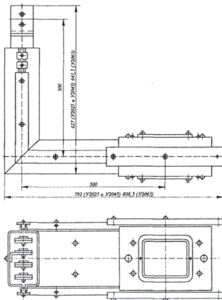
Рис.1.8 Секции угловые горизонтальные правые
