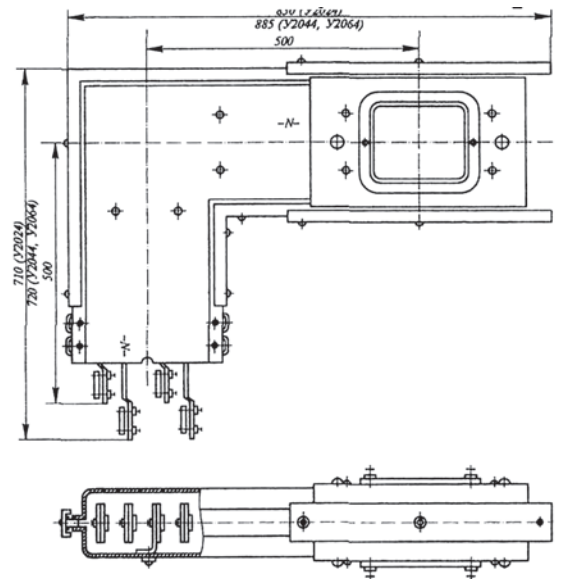
Рис.1.7. Секции угловые вертикальные вниз
